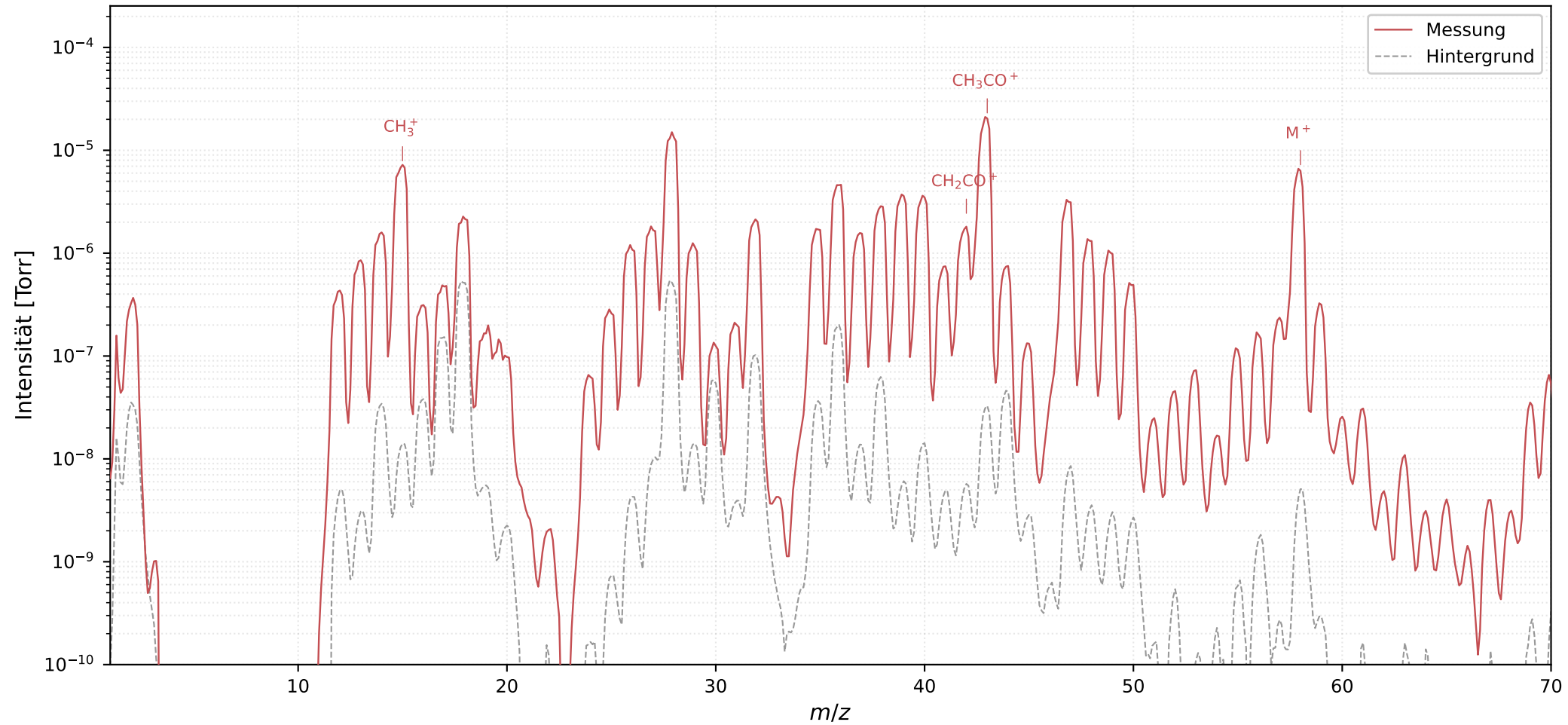
Aceton ( \text{C}_3\text{H}_6\text{O} , M = 58 ) — Messung und Hintergrund (logarithmisch)
